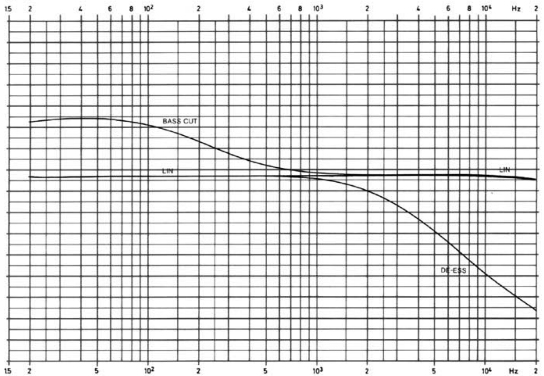
Bass Cut und De-Ess Funktion Bereichsschalter: LIM; Output gain: 0 dB; Comp gain: 0 dB; U_{Ein} : +16 dB
