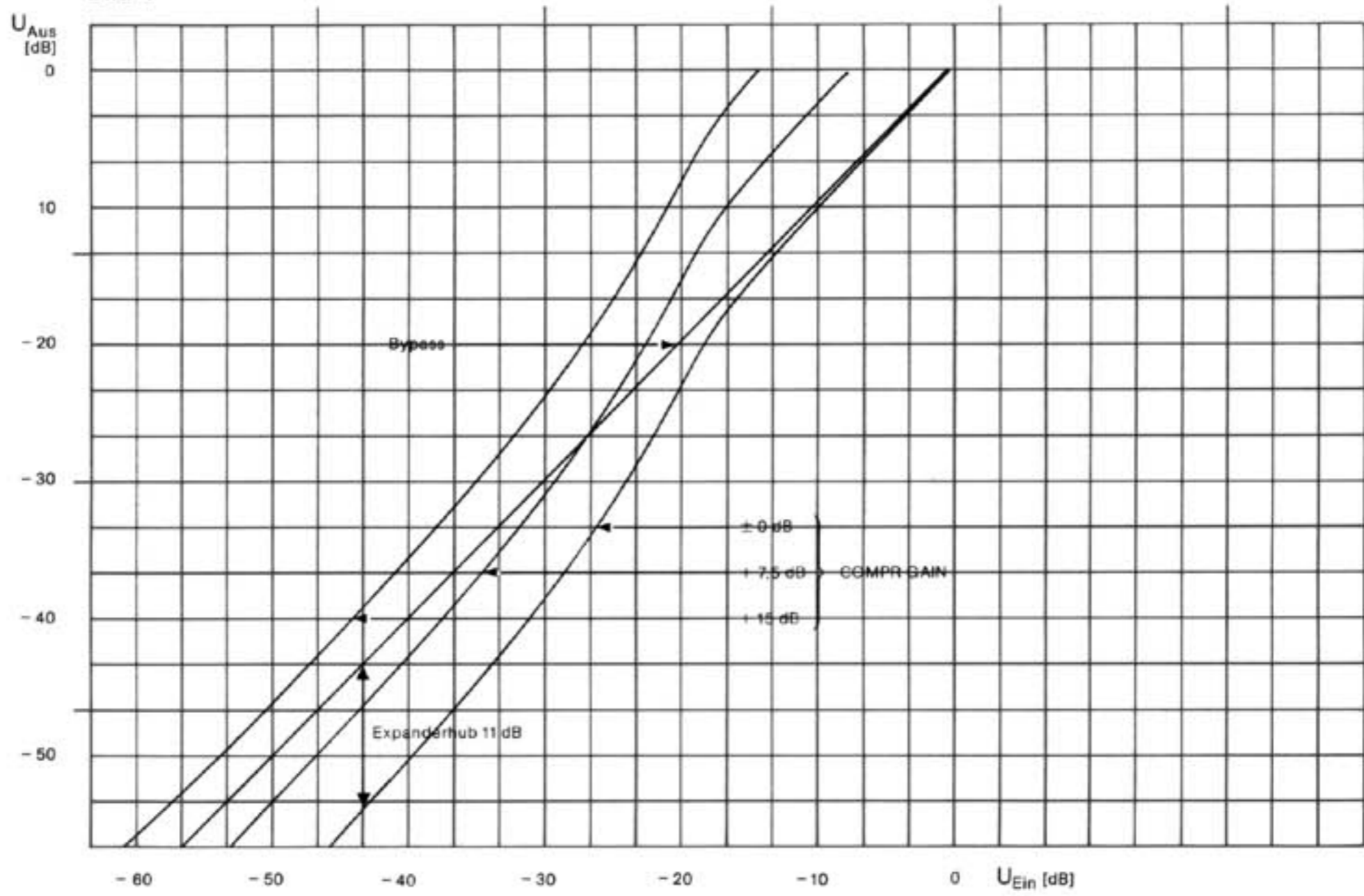
Expanderkennlinie Bereichsschalter Stellung 1:1 Threshold: -20 dB
