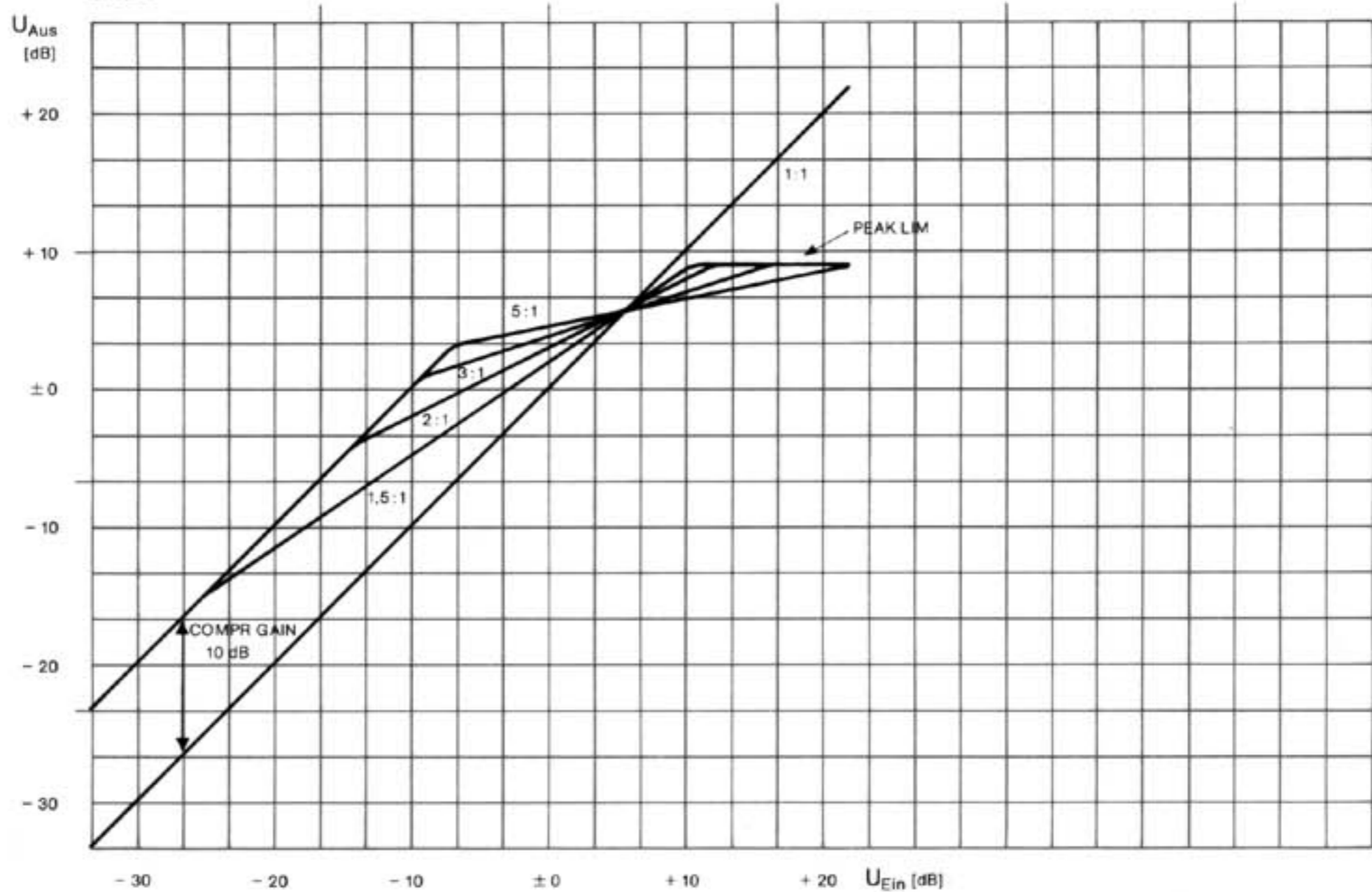
Compressorkennlinie wie Bild 2 Peak Limiter in Funktion Anschlüsse 20-21 am Stecker 1 verbunden
